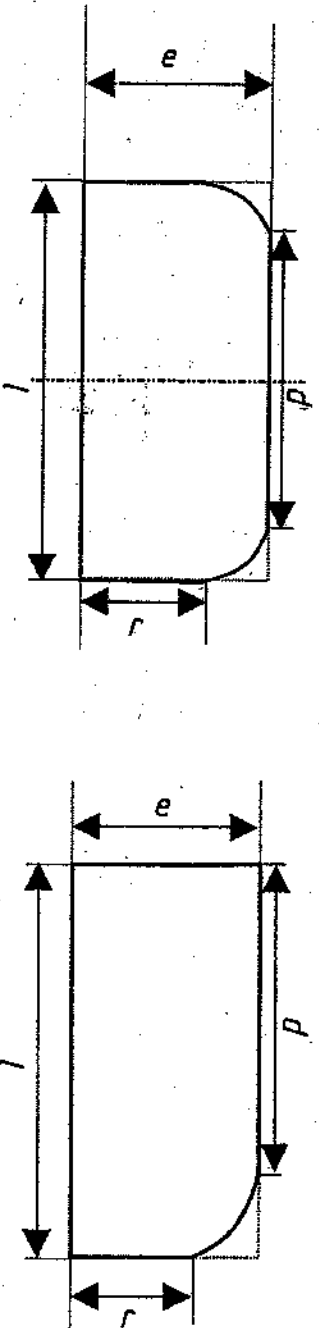
Bild 9 – Höchstzulässige Abmessungen für Rotkern bei Buche
